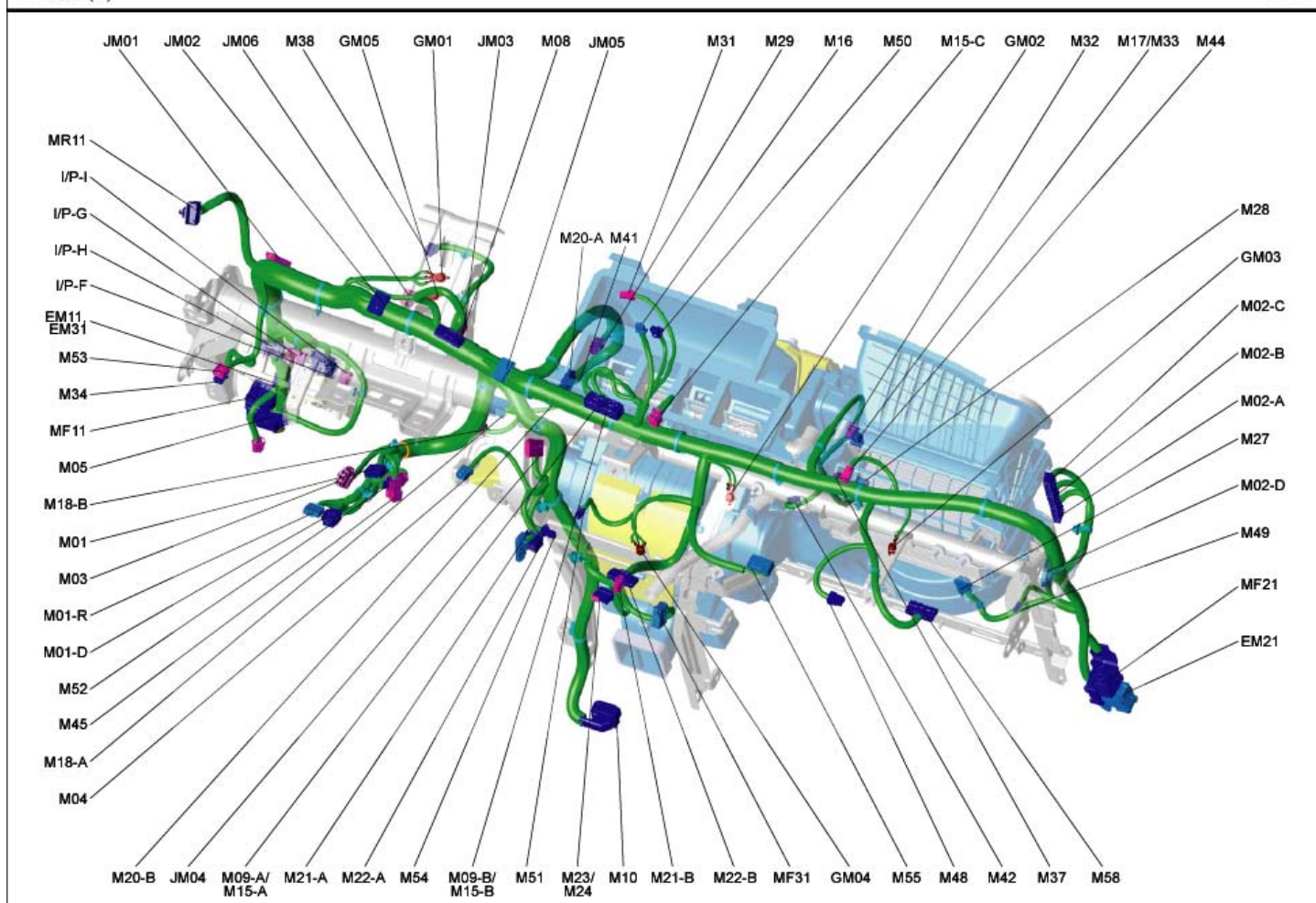
主线束(1)
